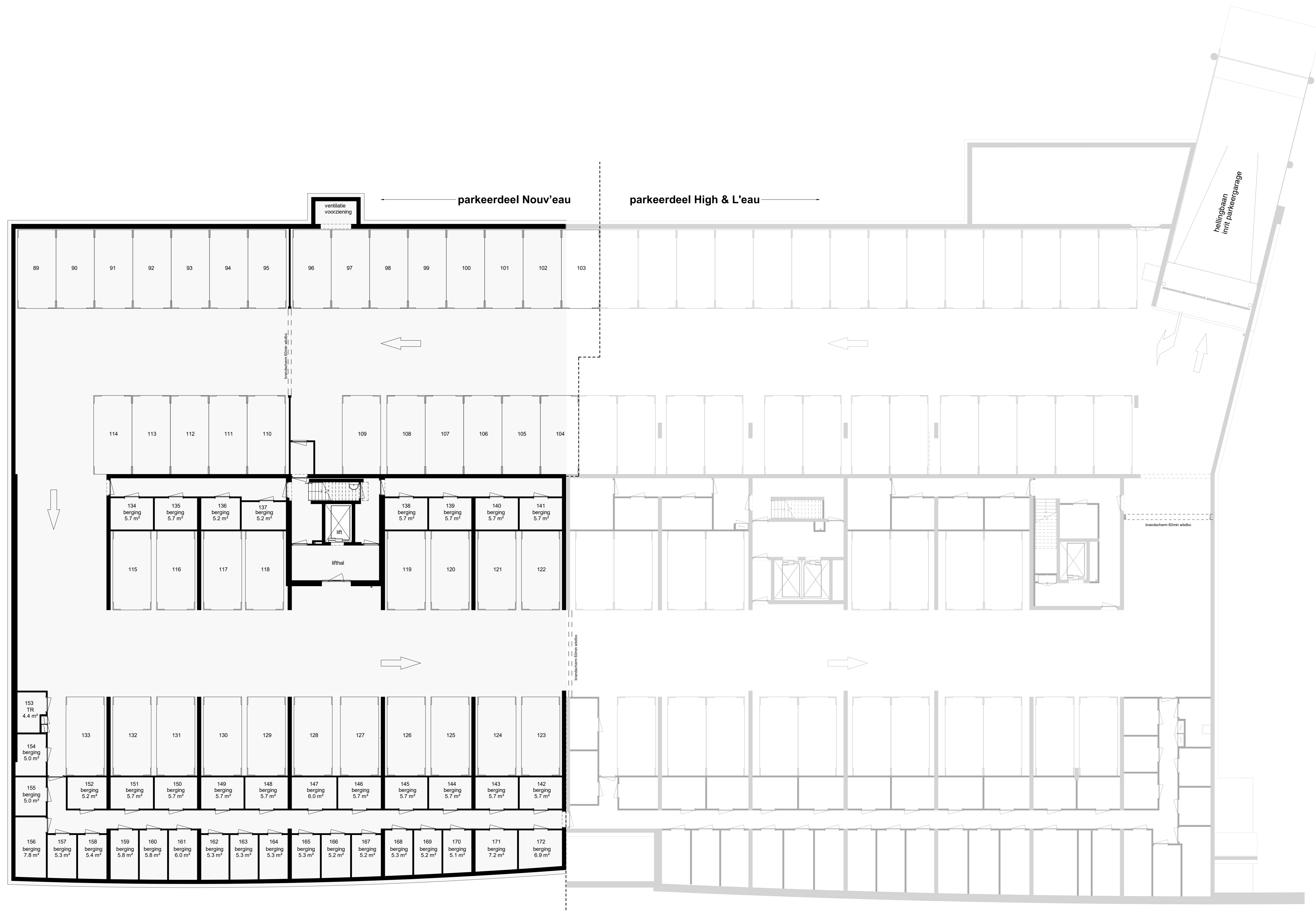
kelderverdieping schaal 1 : 100
