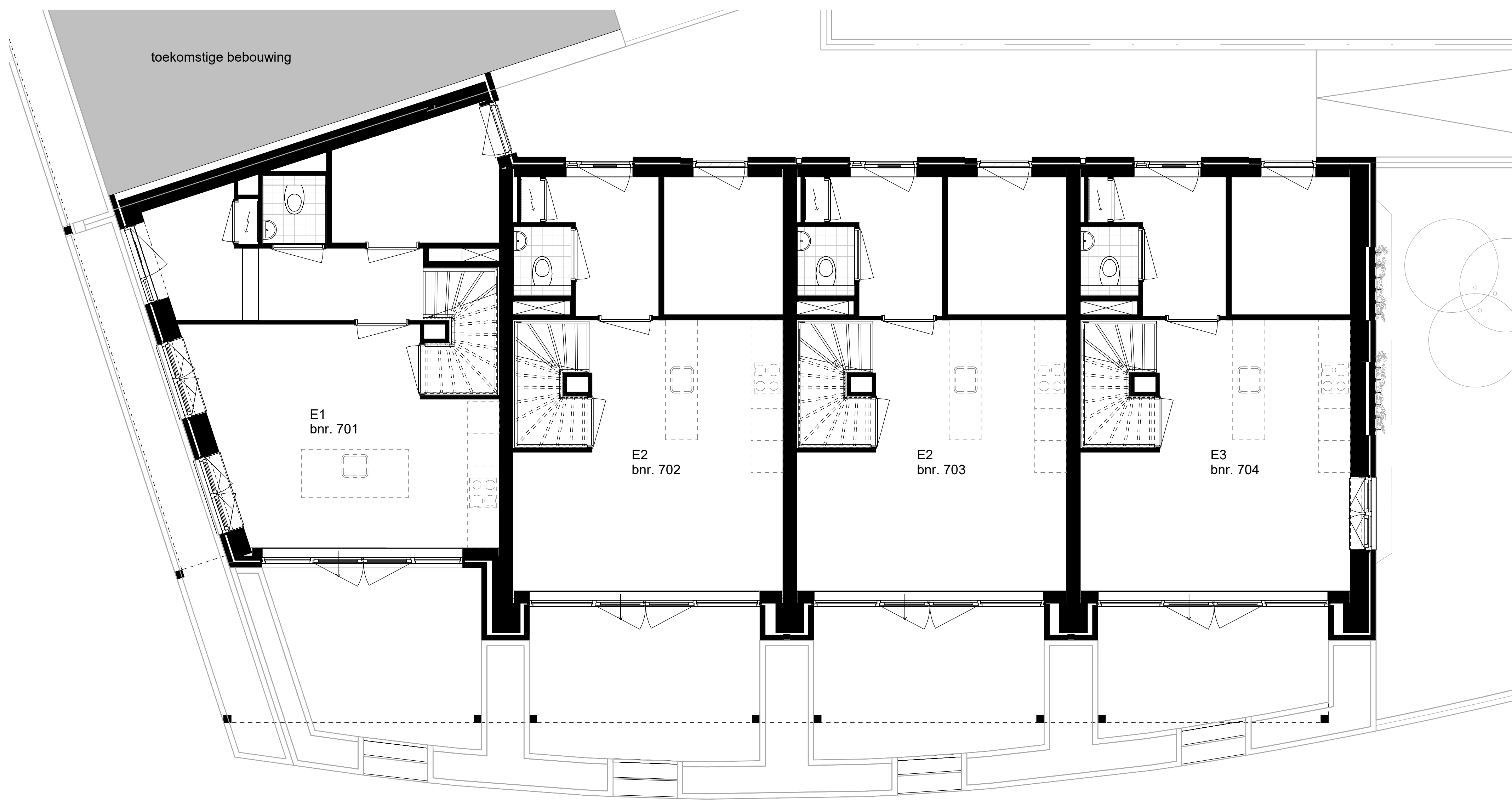
begane grond schaal 1 : 50
