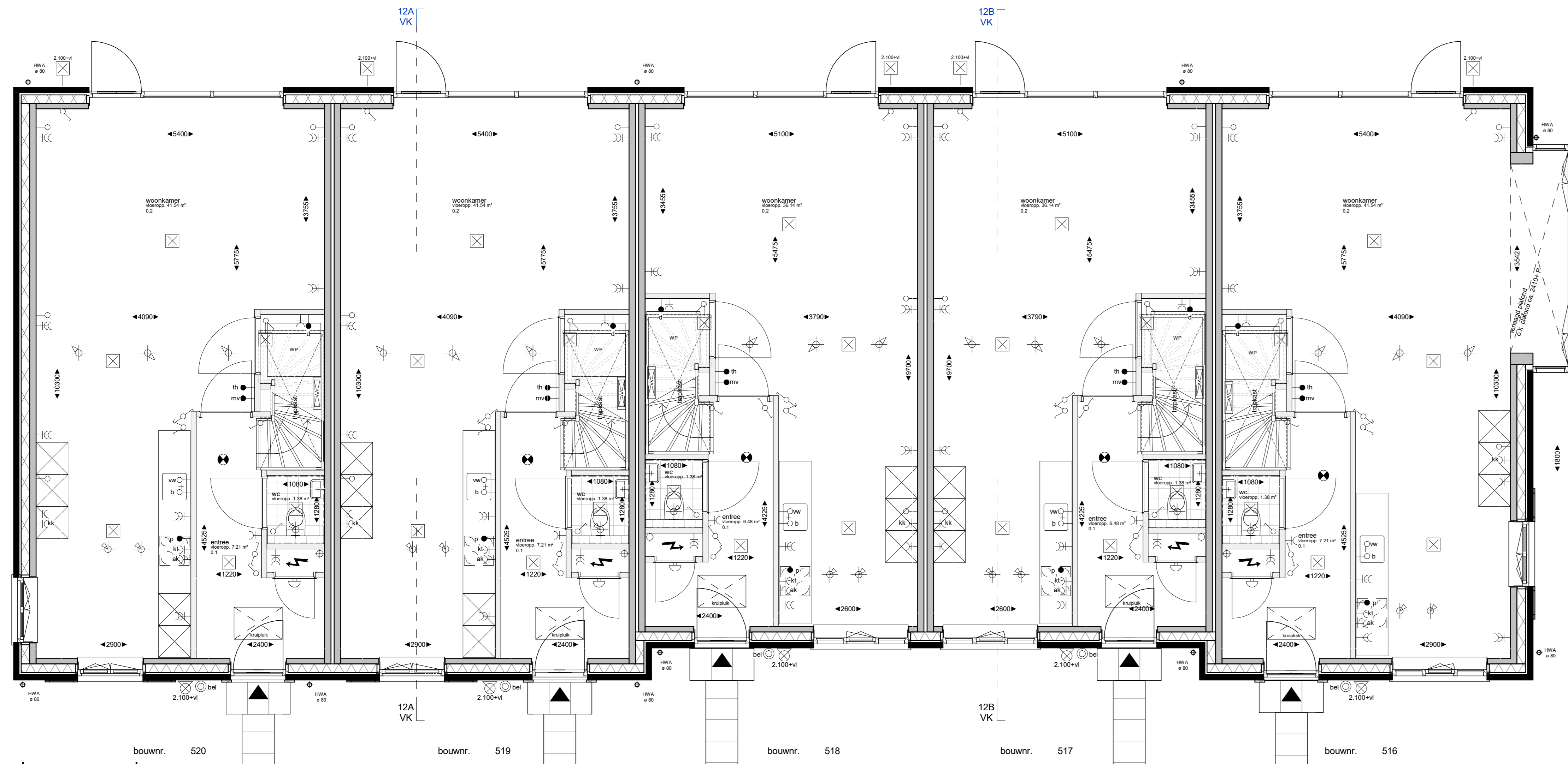
begane grond 1:100
