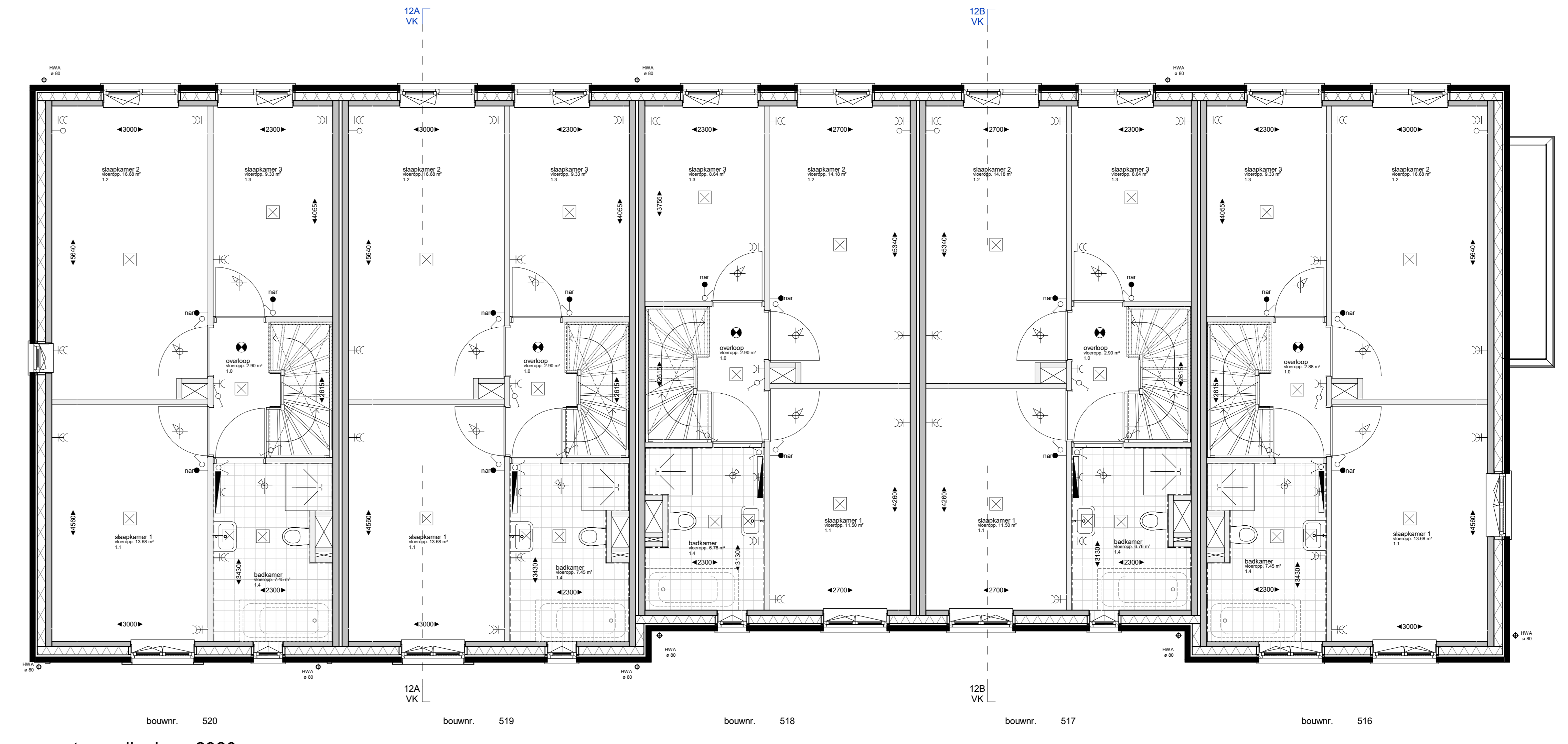
eerste verdieping +2920 1:100
