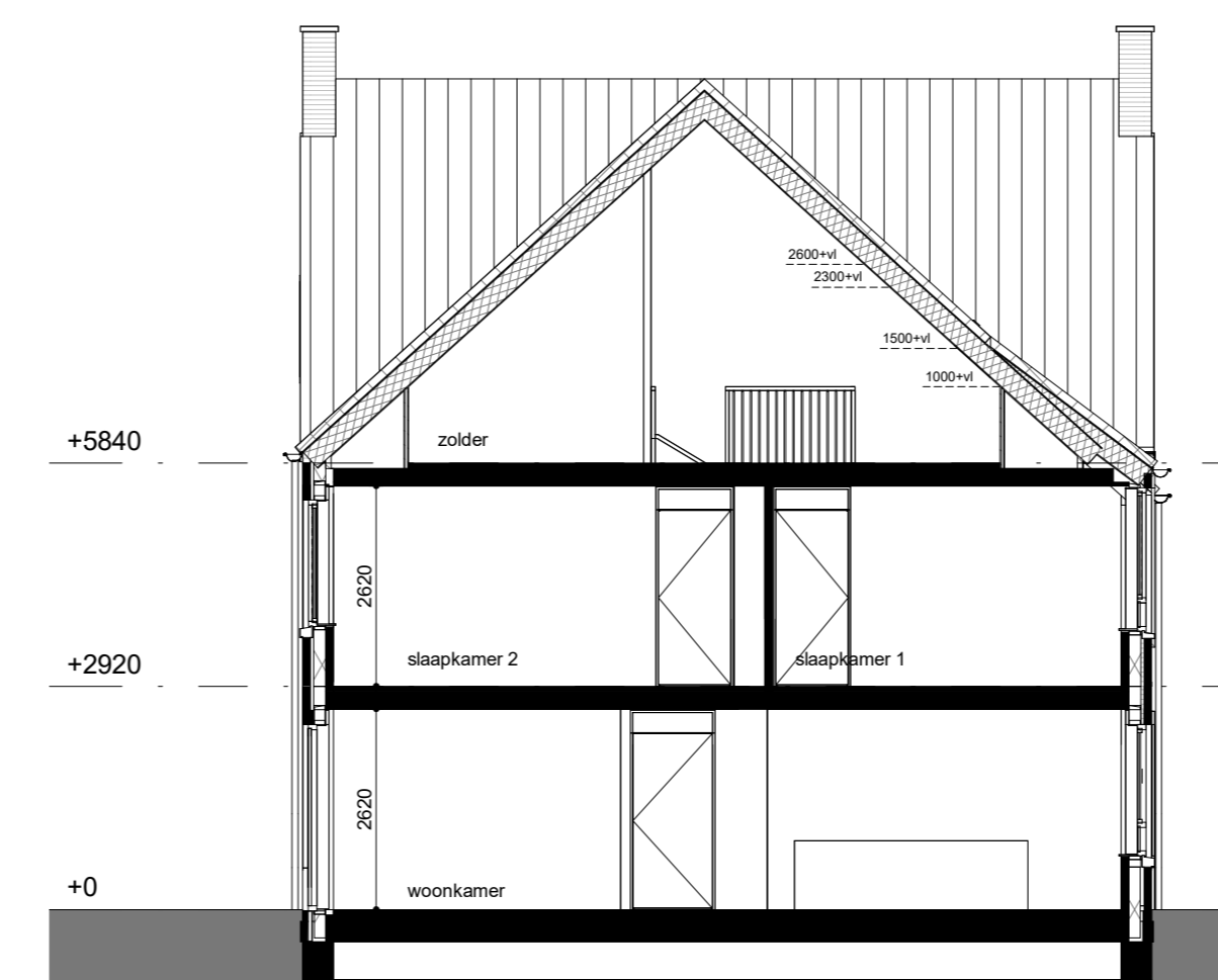
doorsnede 12A 1:100
