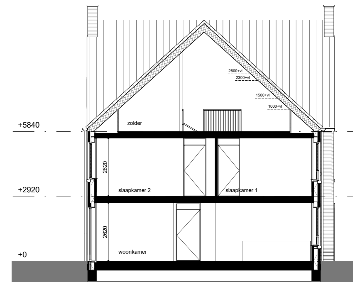
doorsnede 12B 1:100
