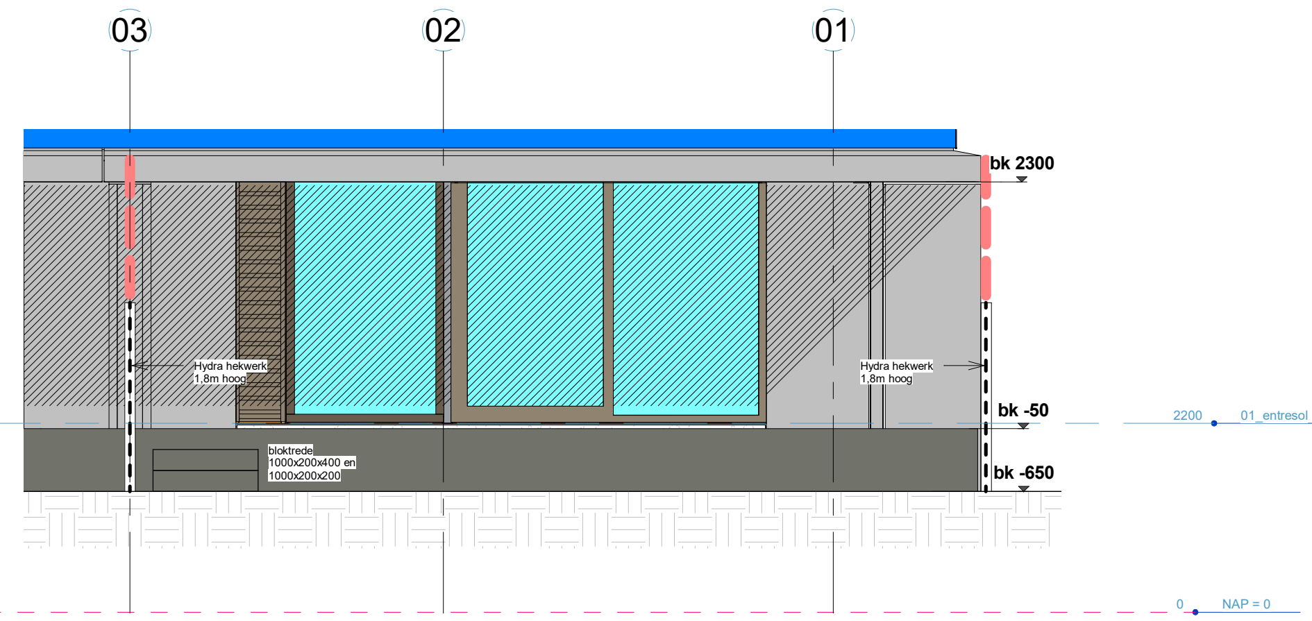
Achtergevel 1:50
