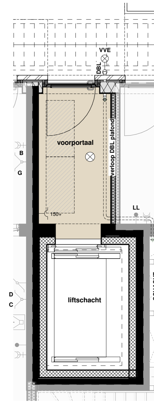
nivo 08, 25.300+P
