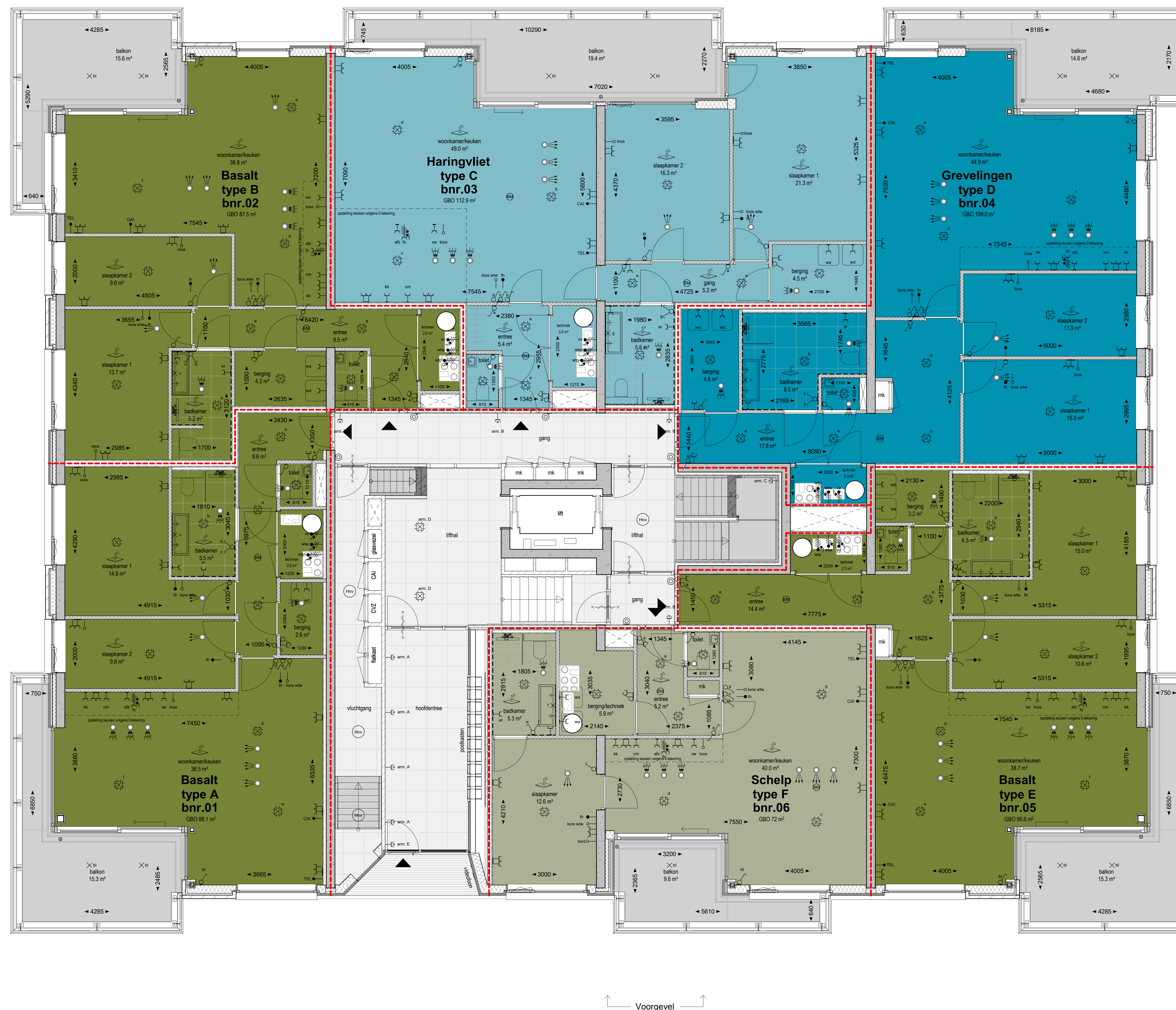
Begane grond gebouw A 1:50
